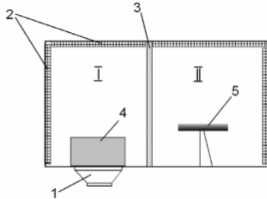
Рис. 4.1. Схема лабораторного стенда БЖ 2
