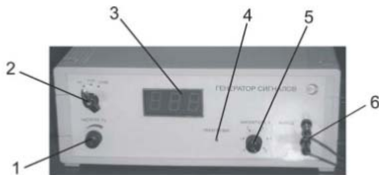
Рис. 4.2. Передняя панель генератора звуковых сигналов
